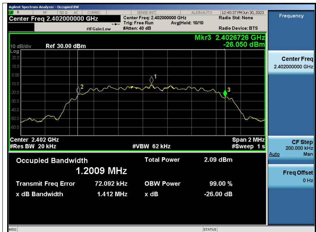
Test_Graph_EDR_2402_2Mbps_OBW
