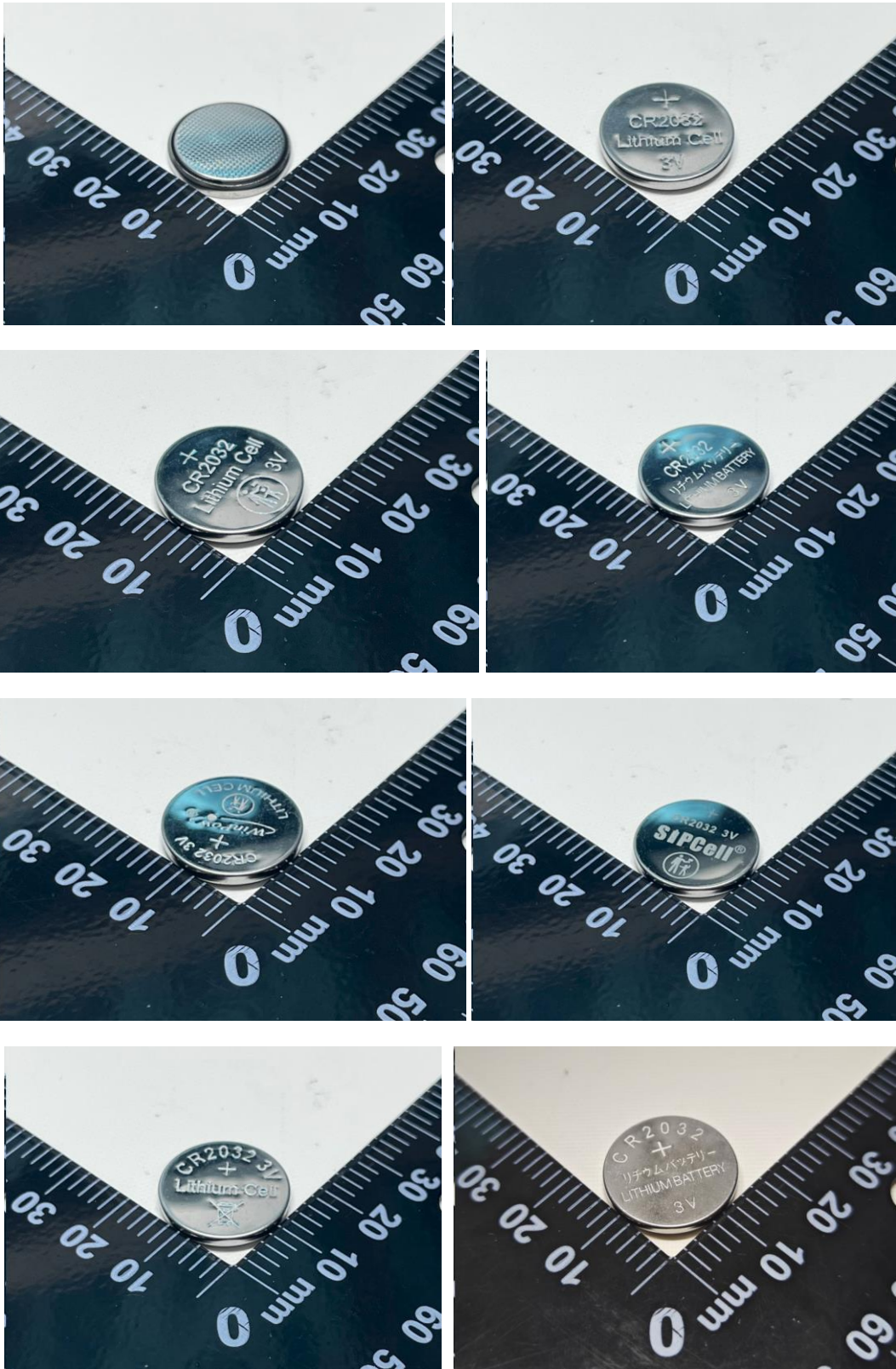
Cell/电芯（CR2032 3V 210mAh）
